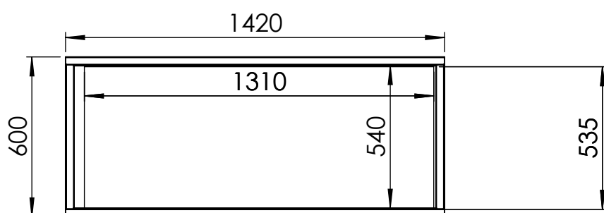
PLANTA
